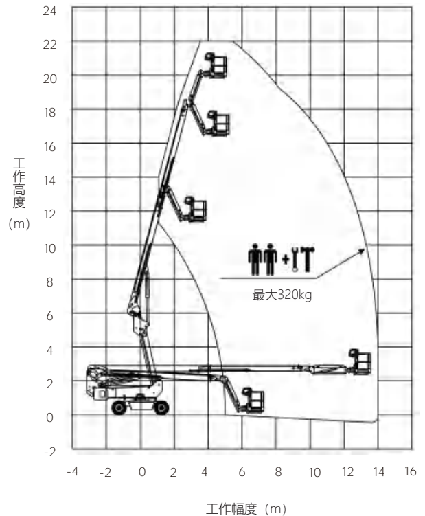
LT20JE -c 性能曲线图
